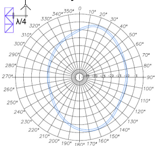
Diagrama Horizontal ajustado Lateral a ¼ espaçamento
