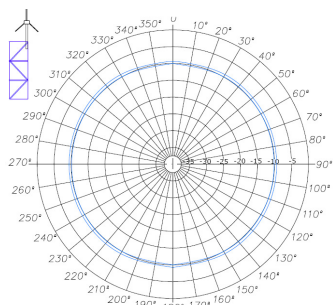
Diagrama Horizontal ajustado Lateral a ¼ espaçamento
